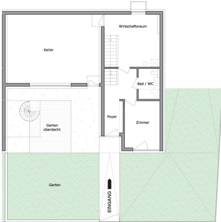
ERDGESCHOSS
